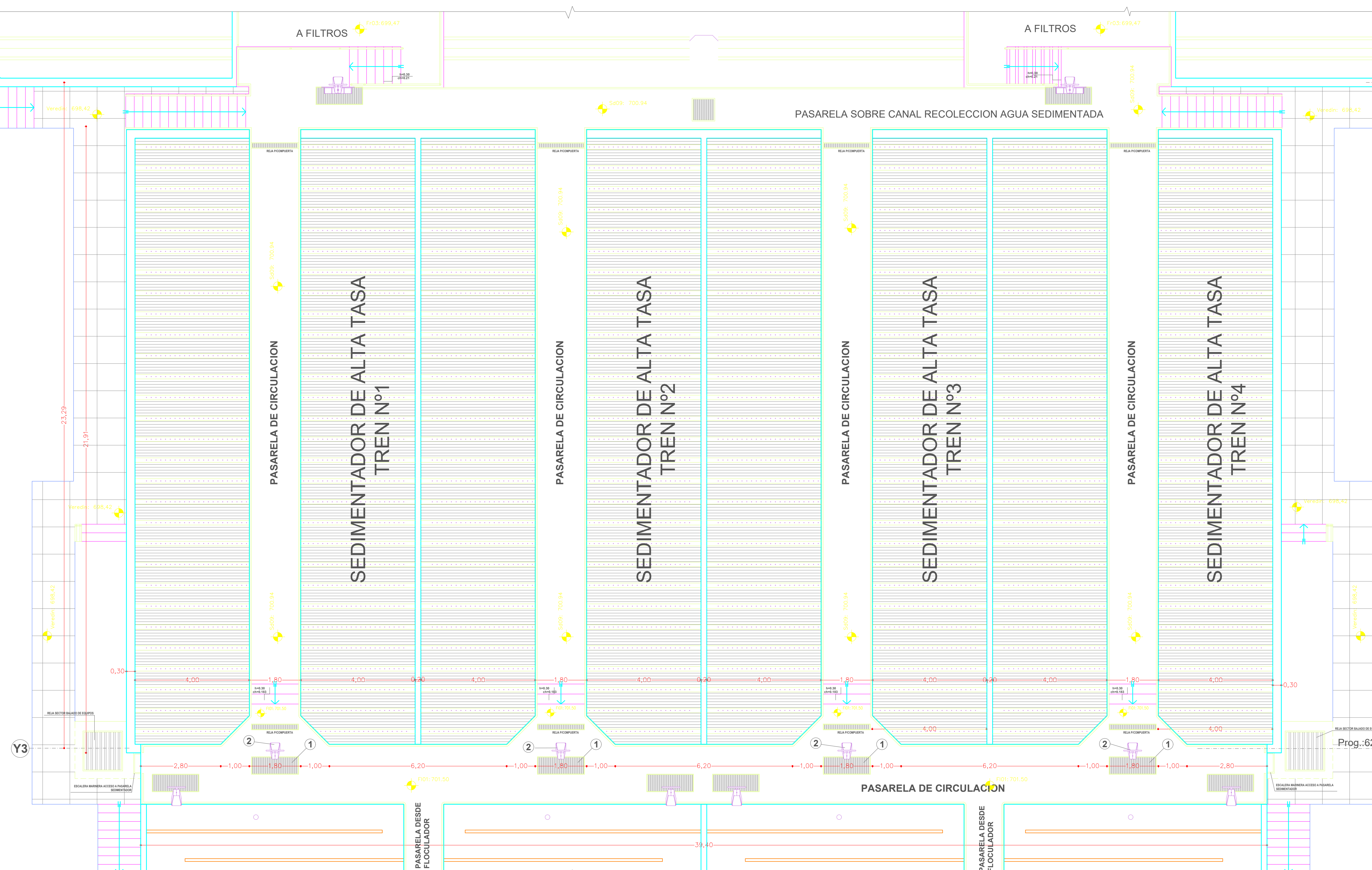
PLANTA P1 NIVEL: 702.50
